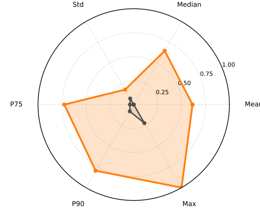
SWEET
