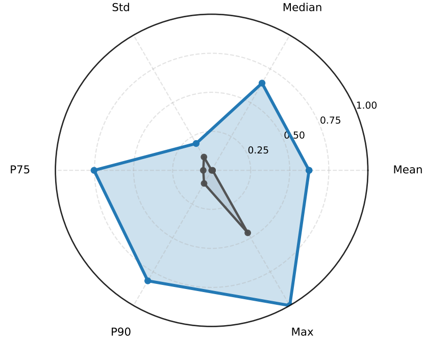
KGW
