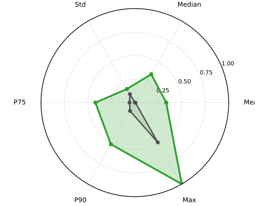
MorphMark
